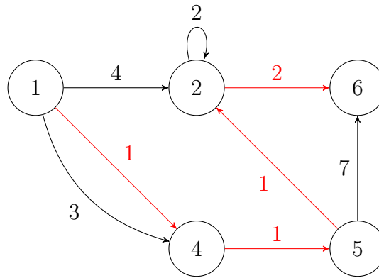
Abbildung 1: Beispielgraph
